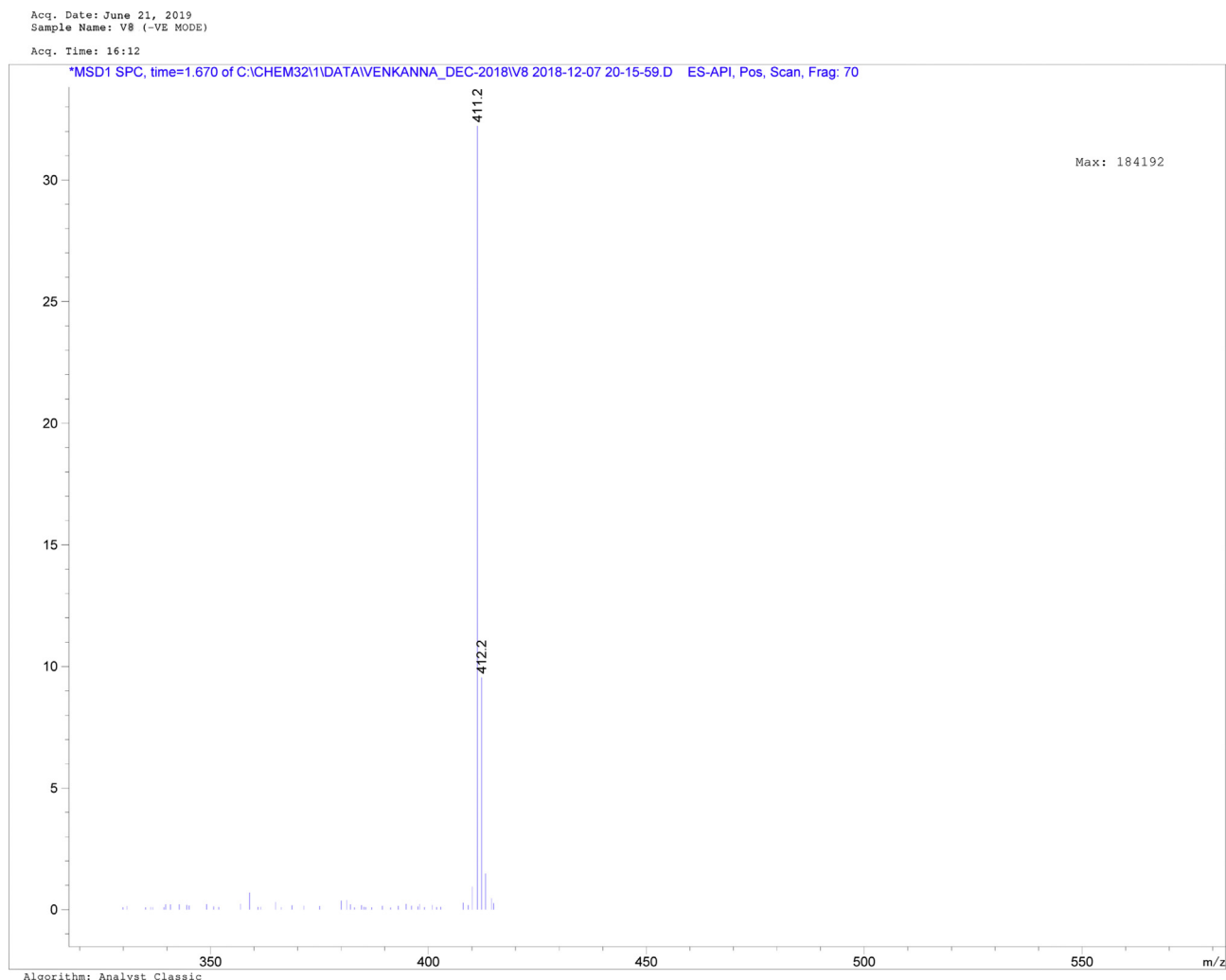
Fig. 18. Mass spectrum of 2, 2'-((propane-1,3-diylbis(azanylylidene))bis(ethan-1-yl-1-ylidene))bis(naphthalen-1-ol).
