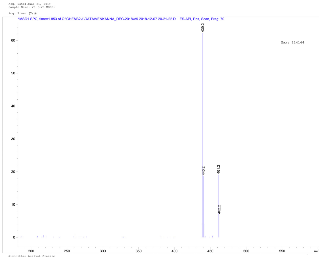
Fig. 20. Mass spectrum of 2, 2'-((pentane-1,3-diylbis(azanylylidene))bis(ethan-1-yl-1-ylidene))bis(naphthalen-1-ol).
