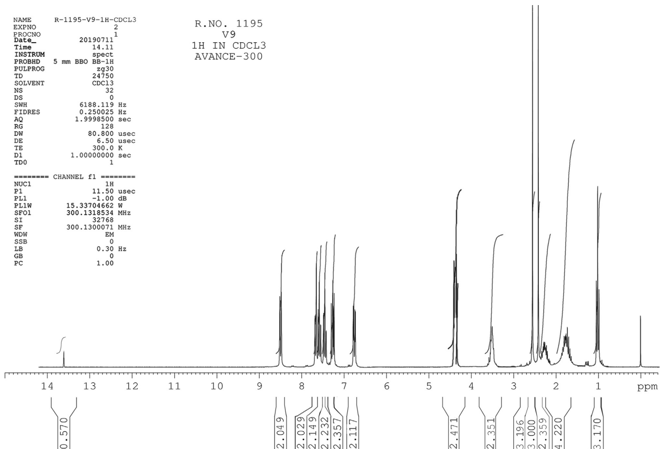
Fig. 12. ^1\text{H} NMR spectrum of 2,2'-((pentane-1,3-diylbis(azanylylidene))bis(ethan-1-yl-1-ylidene))bis(naphthalen-1-ol).
