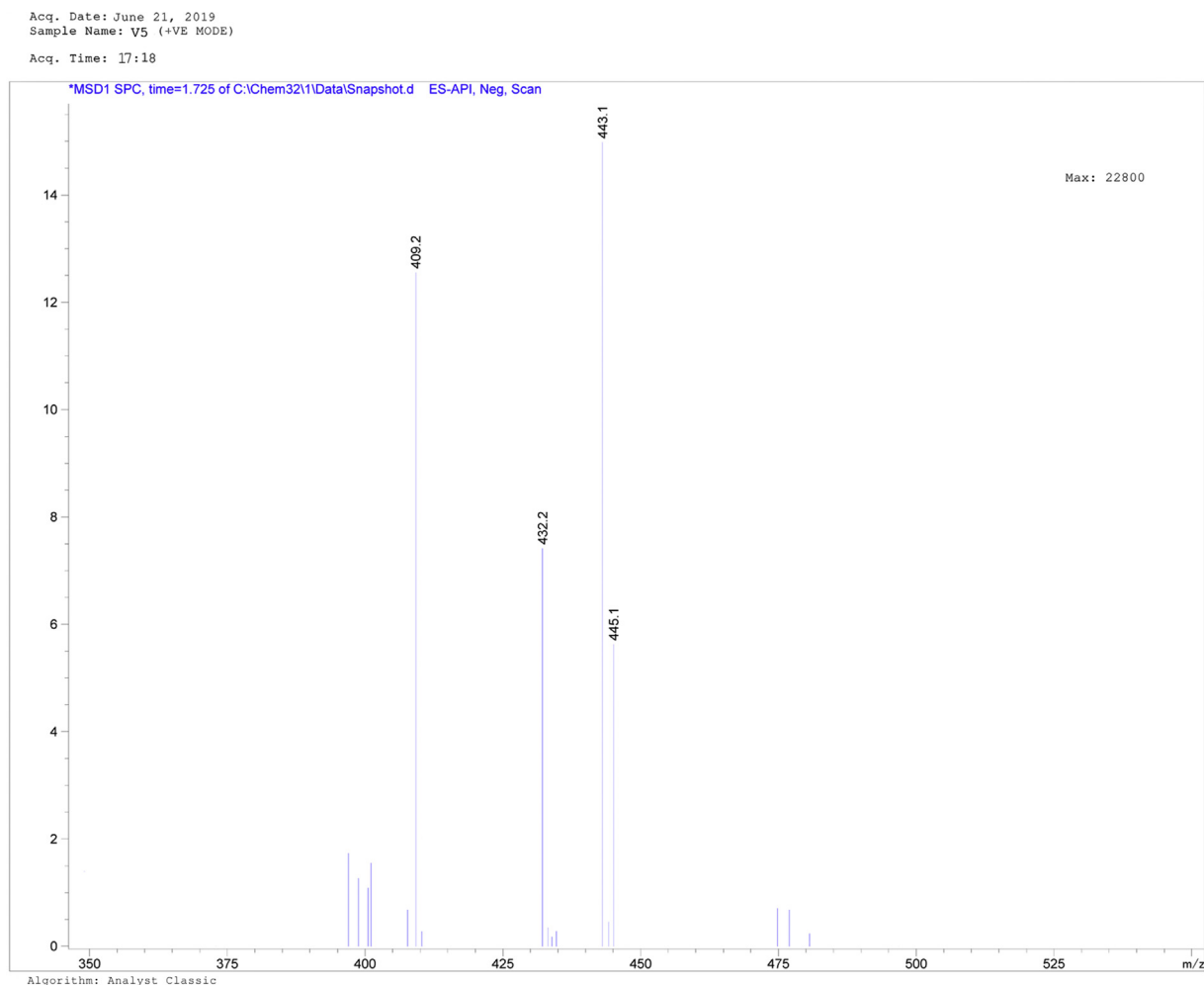
Fig. 19. Mass spectrum of 2,2'-((propane-1,3-diylbis(azanylylidene)))bis(ethan-1-yl-1-ylidene))bis(4-chloronaphthalen-1-ol).
