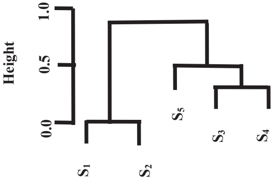
Fig. 3. Dummy dendrogram.
