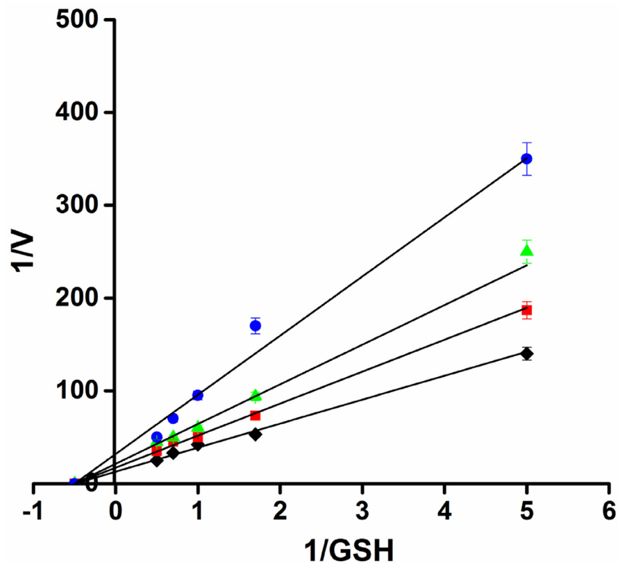
Fig. 6. Dichlorvos K_i values.
