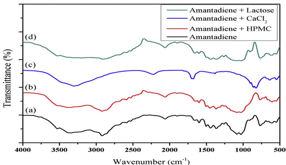
Fig. 6. FTIR spectra for a) Amantadiene, b) Amantadiene + HPMC, c) Amantadiene + \text{CaCl}_2 , d) Amantadiene + Lactose.
