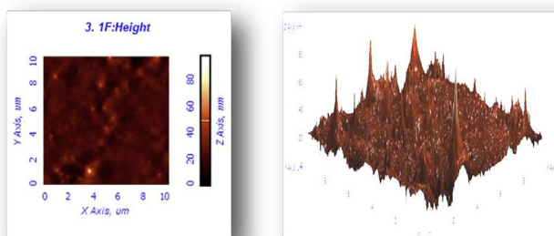
(D) AFM 2D and 3D images of AgNPs of A. marmelos methanolic extract
