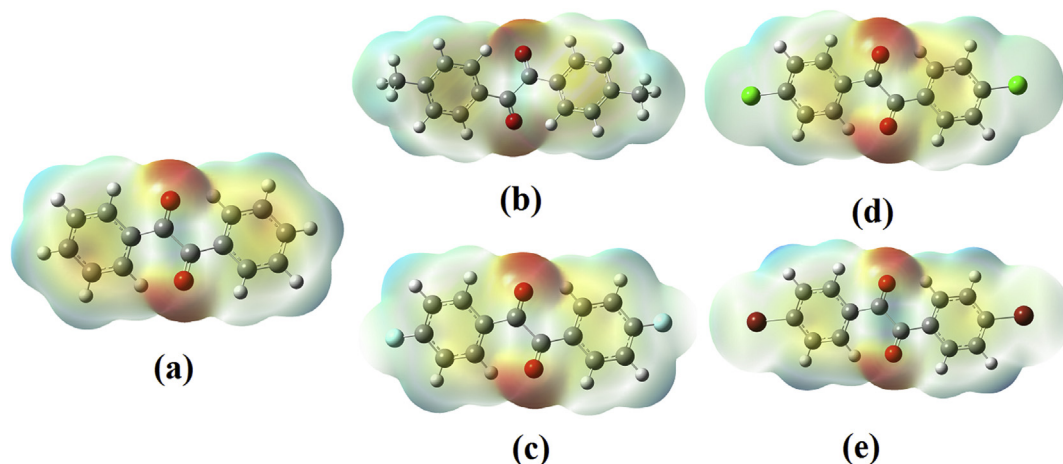
Fig. 4. MEP plots of (a) BZL (b) DMB (c) DFB (d) DCB (e) DBB.
