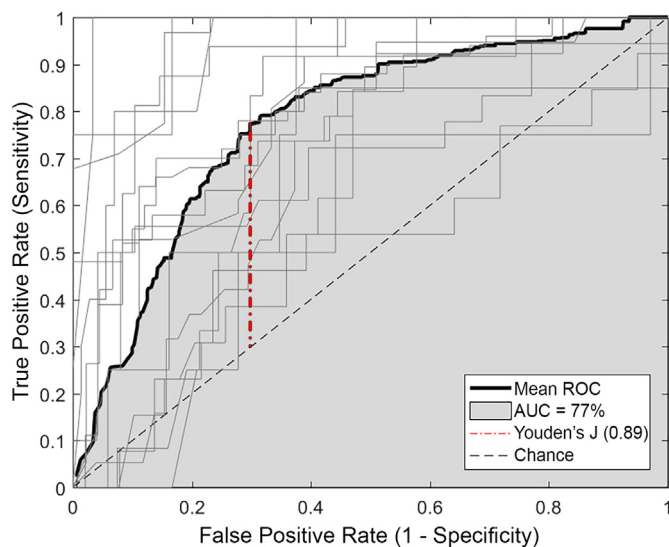
Fig. 3. ROC analysis.
