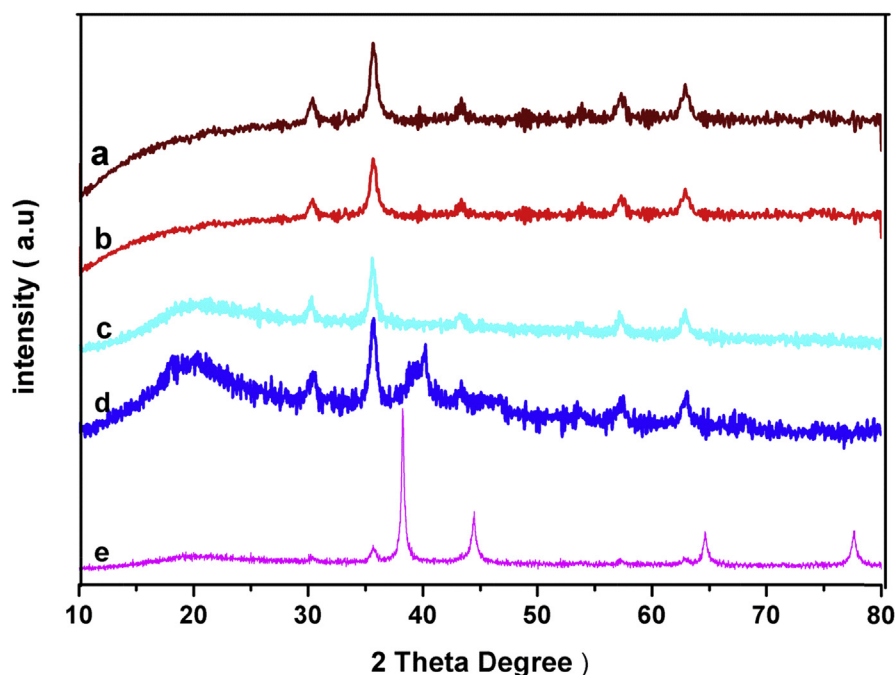
Fig. 2. High angle XRD pattern of (a) \text{Fe}_3\text{O}_4 NPs, (b) \text{Fe}_3\text{O}_4\text{.OANPs} , (c) \text{Fe}_3\text{O}_4\text{-PVBC NPs} , (d) \text{Fe}_3\text{O}_4\text{-PVBC-g-PACNPs} and (e) \text{Fe}_3\text{O}_4\text{-PVBC-g-PAC-AuNPs} catalysts.
